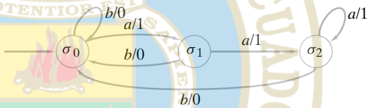
Figura 12.2.1 Diagrama de transición para el ejemplo 12.2.2.
