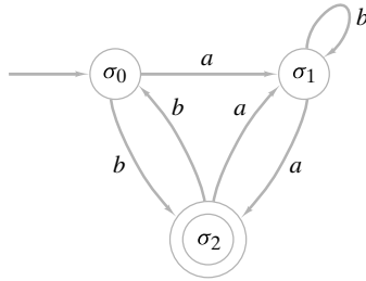
Figura 12.2.3 Autómata de estado finito.
