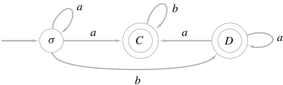
Figura 12.4.3 Diagrama de transición del autómata de estado finito no determinístico del ejemplo 12.4.6.
