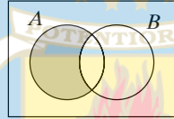
Figura 2.1.4 Un diagrama de Venn de A - B .
