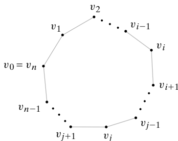
Figura 9.2.3 Ciclo simple.
