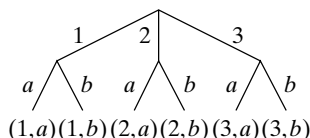
Figura 2.1.7 |X \times Y| = |X| \cdot |Y| , donde X = \{1, 2, 3\} y Y = \{a, b\} .
