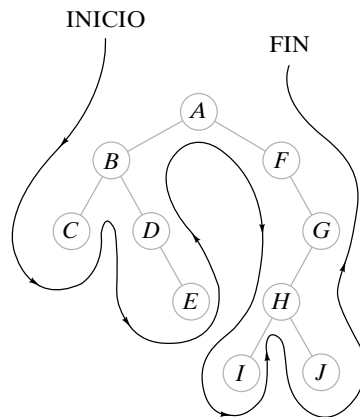
Figura 9.6.5 Recorrido preorden.
