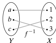
Figura 2.2.12 Inversa de la función en la figura 2.2.11. La inversa se obtiene invirtiendo todas la flechas de la figura 2.2.11. ◀
