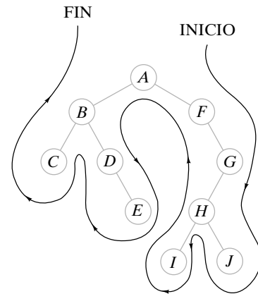
Figura 9.6.6 Recorrido postorden en reversa.
