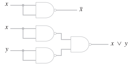
Figura 11.5.3 Circuitos combinacionales usando sólo compuertas NAND que calculan \bar{x} y x \vee y .
