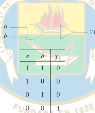
Figura 11.2.4 Un circuito combinatorio y su tabla lógica.
