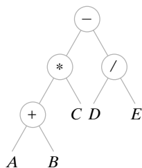
Figura 9.6.7
