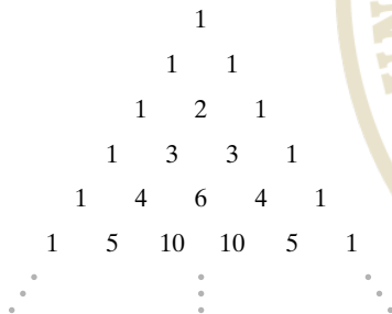
Figura 6.7.1 Triángulo de Pascal.
