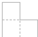
Figura 1.7.3 Un tromino.
