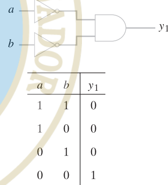
Figura 11.2.5 Circuito combinatorio y su tabla lógica, que es idéntica a la tabla lógica de la figura 11.2.4. Se dice que los circuitos de las figuras 11.2.4 y 11.2.5 son equivalentes porque tienen tablas lógicas idénticas.
