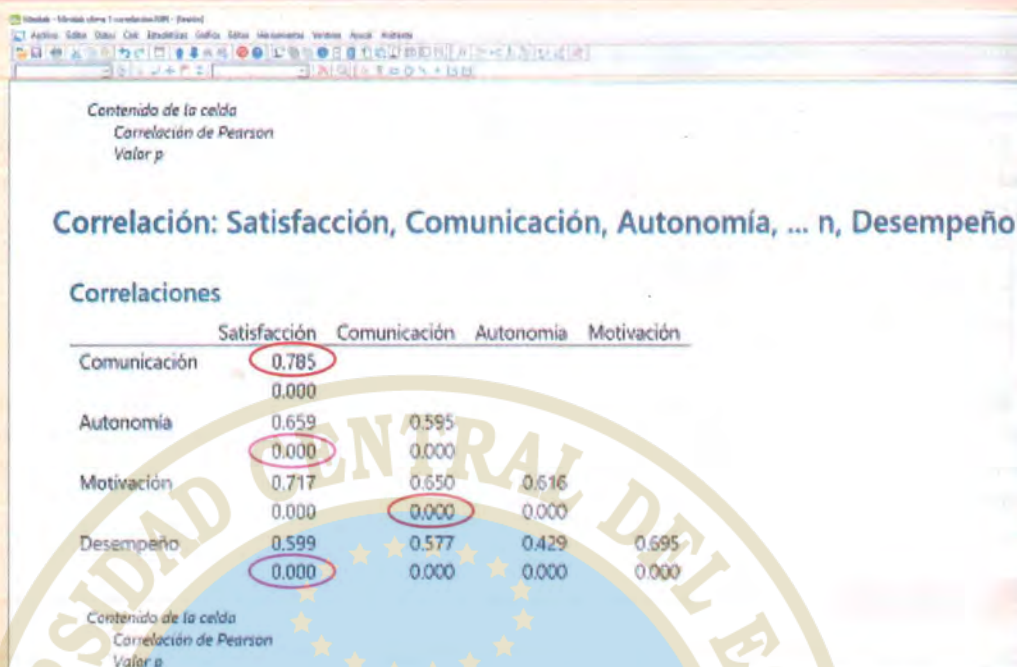
Figura 10.20. Ejemplo de matriz de correlaciones en Minitab®.
