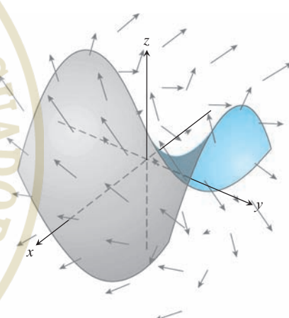
FIGURA 16.9 Una superficie, como una red o un paracaídas, en un campo vectorial que representa los vectores velocidad del flujo de agua o aire. Las flechas muestran la dirección y sus longitudes indican la rapidez.
