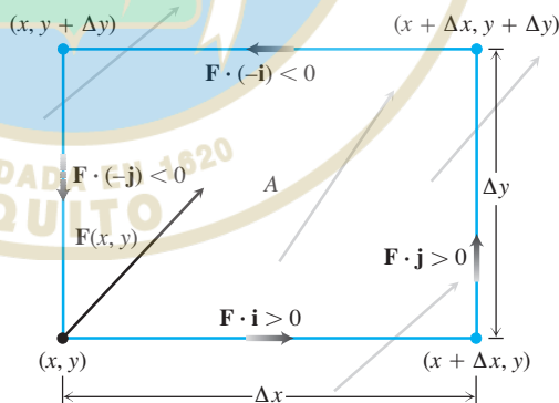
FIGURA 16.29 La tasa a la que el fluido fluye a través del rectángulo A por la orilla inferior en la dirección \mathbf{i} es aproximadamente \mathbf{F}(x, y) \cdot \mathbf{i} \Delta x , la cual es positiva para el campo vectorial \mathbf{F} mostrado aquí. Para aproximar la tasa de circulación en el punto (x, y) , calculamos las tasas (aproximadas) del flujo a través de cada orilla en la dirección de las flechas sombreadas, sumamos esas tasas, y luego dividimos la suma entre el área de A . Al tomar el límite como \Delta x \rightarrow 0 y \Delta y \rightarrow 0 obtenemos la tasa de circulación por unidad de área.
