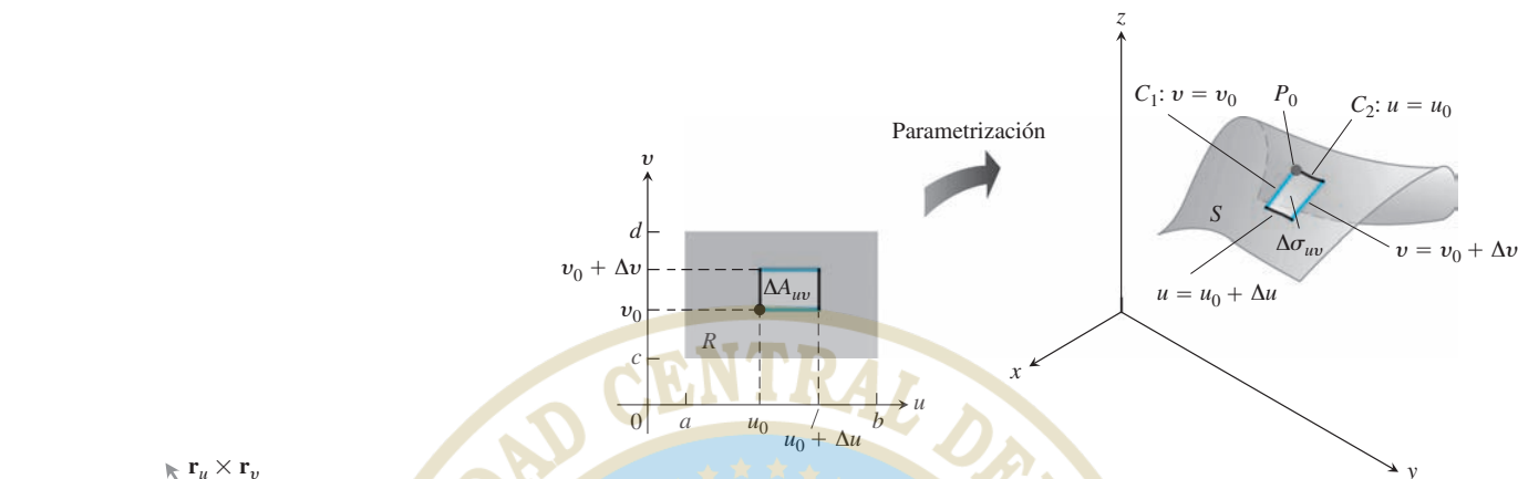
FIGURA 16.41 Un elemento de área rectangular \Delta A_{uv} en el plano uv se convierte en un elemento de área curvado \Delta \sigma_{uv} sobre S .
