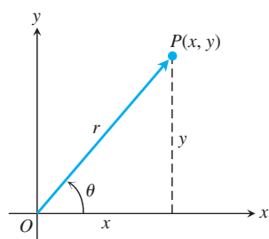
FIGURA A.24 Este diagrama de Argand representa a z = x + iy como un punto P(x, y) y como un vector \overrightarrow{OP} .
