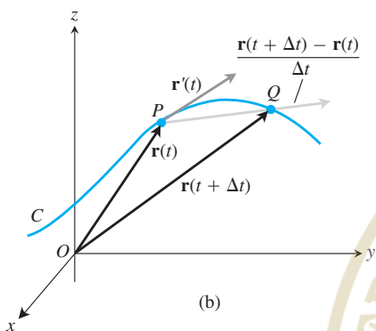
FIGURA 13.5 Cuando \Delta t \rightarrow 0 , el punto Q se aproxima al punto P a lo largo de la curva C . En el límite, el vector \overrightarrow{PQ}/\Delta t se convierte en el vector tangente \mathbf{r}'(t) .
