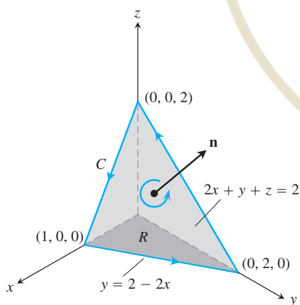
FIGURA 16.62 La superficie plana del ejemplo 7.
