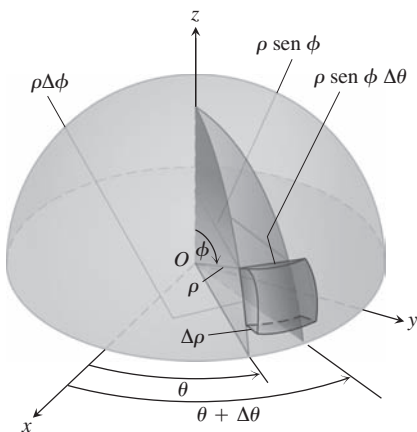
FIGURA 15.51 En coordenadas esféricas, dV = d\rho \cdot \rho \, d\phi \cdot \rho \sin \phi \, d\theta = \rho^2 \sin \phi \, d\rho \, d\phi \, d\theta.
