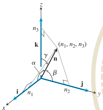
FIGURA 16.70 Los componentes de \mathbf{n} son los cosenos de los ángulos \alpha , \beta y \gamma que forma con \mathbf{i} , \mathbf{j} y \mathbf{k} .
