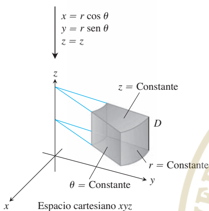
FIGURA 15.60 Las ecuaciones x = r \cos \theta , y = r \sin \theta y z = z transforman el cubo G en una cuña cilíndrica D .
