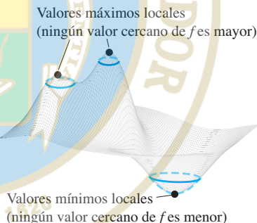
FIGURA 14.40 Un máximo local es un pico de montaña y un mínimo local es el fondo de un valle.
