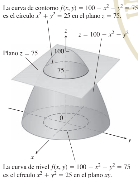
FIGURA 14.6 Un plano z = c paralelo al plano xy que corta una superficie z = f(x, y) produce una curva de contorno.
