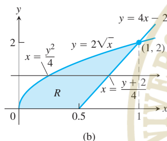
FIGURA 15.18 (a) La región sólida “como cuña”, cuyo volumen se obtuvo en el ejemplo 4. (b) La región de integración R que muestra el orden dx dy .
