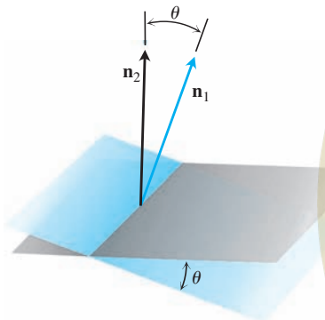
FIGURA 12.42 El ángulo entre dos planos se obtiene a partir del ángulo entre sus normales.
