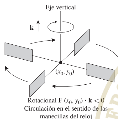
FIGURA 16.30 En el flujo de un fluido incompresible sobre una región plana, el componente \mathbf{k} del rotacional mide la tasa de giro del fluido en un punto. El componente \mathbf{k} del rotacional es positivo en los puntos donde la rotación va en sentido contrario al de las manecillas del reloj y negativo donde la rotación es en el sentido de las manecillas.
