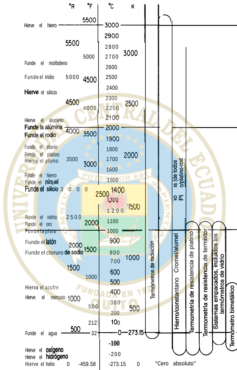
Figura 1.4 Los instrumentos para medir la temperatura abarcan el intervalo desde cerca del cero absoluto hasta más allá de 3000 K. El diagrama indica los métodos preferidos de instrumentación térmica para las distintas regiones de temperatura.
