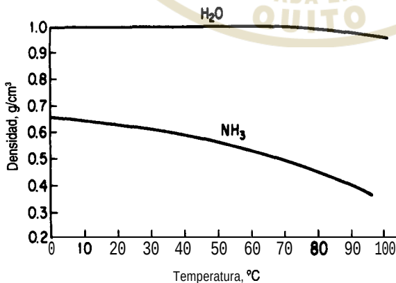
Figura 1.1 Densidades del H 2 O y NH 3 líquidos en función de la temperatura.
