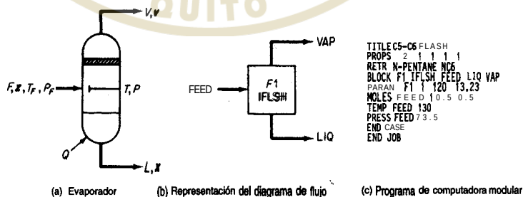
Figura 6.6 Módulo que representa un evaporador instantáneo. (De J. D. Seader, W. D. Seider y A. C. Pauls, Flowtran Simulation—An Introduction , Austin, TX: CACHE, 1987.)
