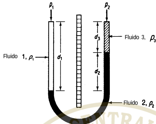
Figura 1.13 Manómetro con tres fluidos.
