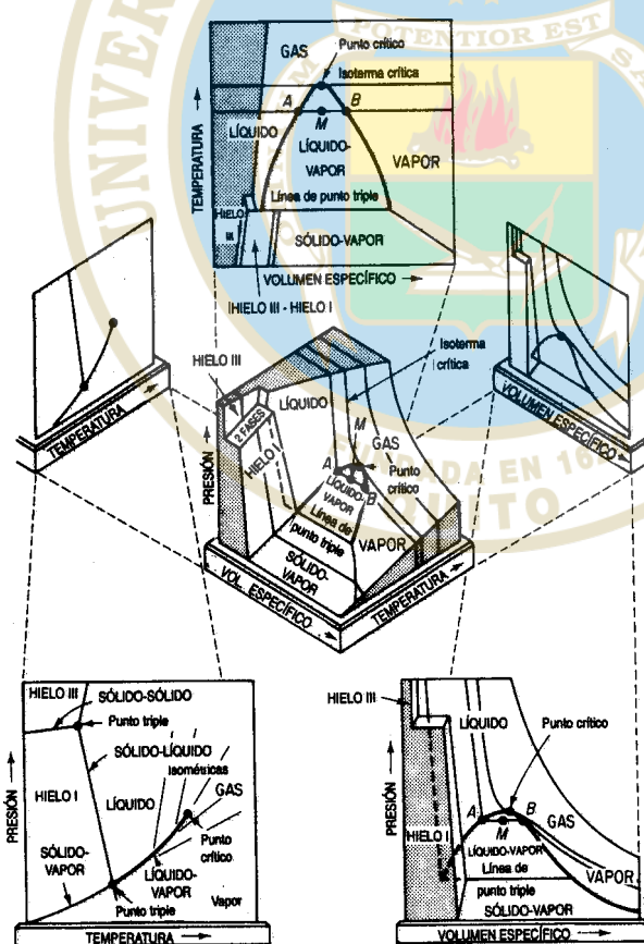
Figura 4.10 Superficie p, \hat{V}, T y proyecciones para H_2O .
