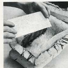
11. Se pone encima y se aprieta contra la resina un «mat» de fibra cortada basto, previamente impregnado en resina.
