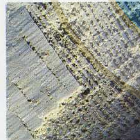
8. Para quitar las marcas de la uña y para definir la forma acabada de la talla se usa el cincel chato.
