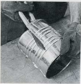
Corte y enderezamiento de una lata de hojalata 1. Se quita la parte de arriba y la de abajo y se corta a lo largo de un lado de la junta con una tijera de hojalatero.
