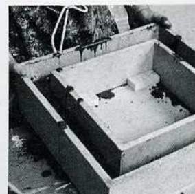
3. Se hace saltar el molde repetidamente sobre la superficie del banco de trabajo para que el hormigón se asiente y se extienda por igual.
