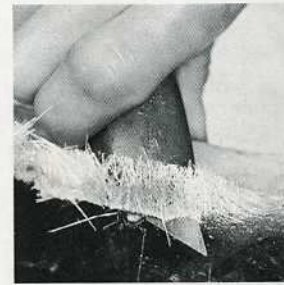
12. Se deja endurecer ligeramente la resina. Con un cuchillo afilado se recorta el «mat» que asome por encima del borde del molde.
