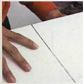
Corte y unión del poliestireno expandido 1. Marcar el bloque con un rotulador y cortar a lo largo de la marca con un cortador de alambre caliente.
