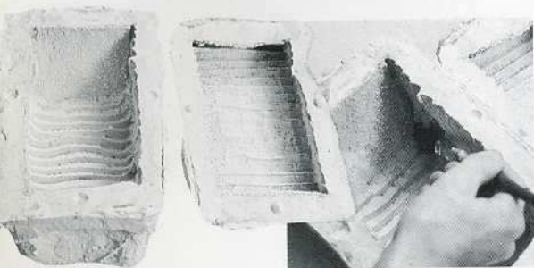
Vaciado de resina en un molde de yeso de un solo uso 1. Lo primero de todo es proteger las manos con una crema aislante. Se trabaja sobre ambas mitades del molde en la forma siguiente:
