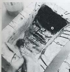
10. Se cataliza resina para estratificados y se aplica a pincel para impregnar el «mat». Se eliminan las burbujas de aire que pueda haber en la resina.
