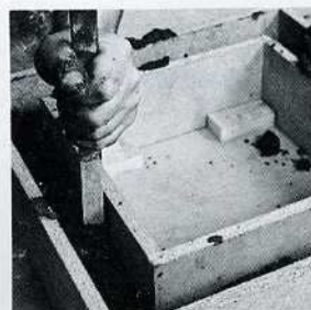
2. Se echa en el molde una capa de mezcla de hormigón espesa y se pudela con una vara o listón para que no se hagan burbujas de aire.
