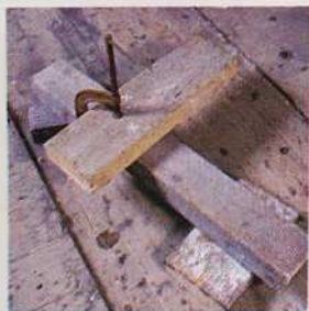
Ensambladura de dos bloques con pernos 1. Se colocan los bloques en la posición adecuada, levantados del suelo y firmemente sujetos unidos con gatos.
