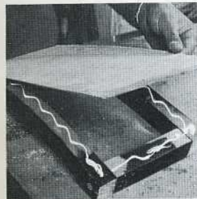
Revestido Para cubrir una estructura de madera pueden usarse paneles de chapa o de madera contrachapada, que también pueden adaptarse a formas curvas. Se encola la estructura y se coloca el panel ajustándolo a aquélla; se asegura con puntas clavadas.
