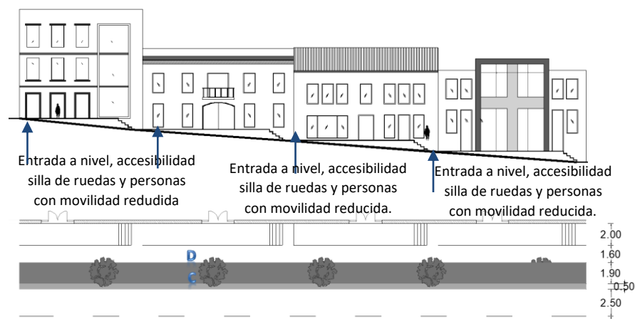
Gráfico 71: esquema en donde se puede apreciar la utilidad de la franja de borde para resolver los desniveles y acceso a las edificaciones, manteniendo la franja de circulación sin interrupciones, en el mismo plano de pendiente
