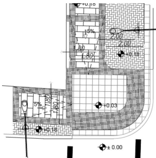
Gráfico 64: rampas antes de llegar a la esquina
