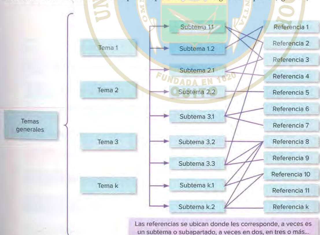
Figura 4.7. Ilustración del proceso de vertebración del índice del marco teórico y ubicación de referencias.
