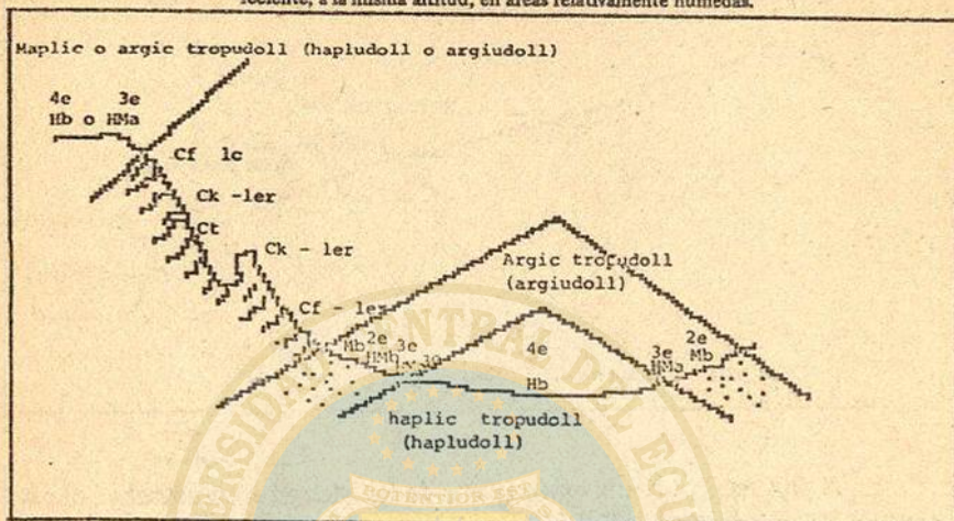
FIGURA No. 2 Asociación de suelos formados de cangahua con suelos formados de ceniza volcánica reciente, a la misma altitud, en áreas relativamente húmedas.
