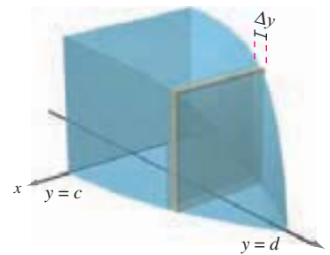
b) Secciones transversales perpendiculares al eje y
