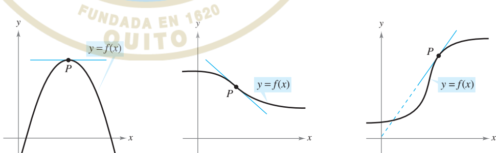
Recta tangente a una curva en un punto Figura 2.2
