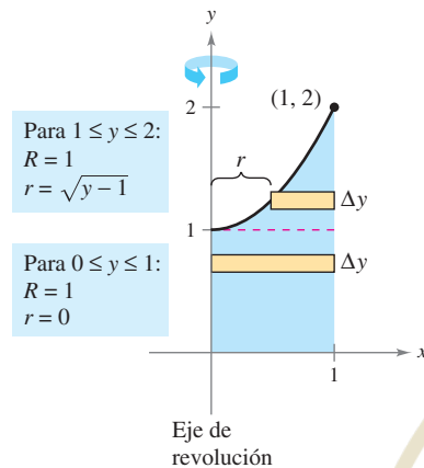
a) Método de los discos
