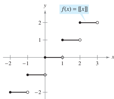
Función parte entera o mayor entero Figura 1.30
