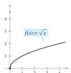
Función raíz cuadrada
