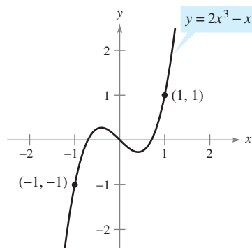
Simetría con respecto al origen Figura P.8
