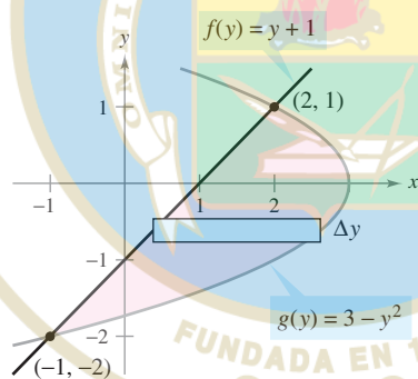
Rectángulos horizontales (integración con respecto a y )
