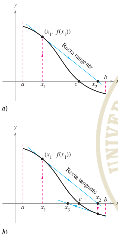
La intersección con el eje x de la recta tangente se aproxima a cero de f
