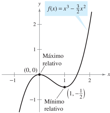
Extremos relativos de f Figura 3.18
