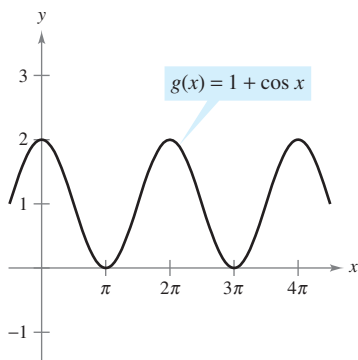
b) Función par Figura P.31
