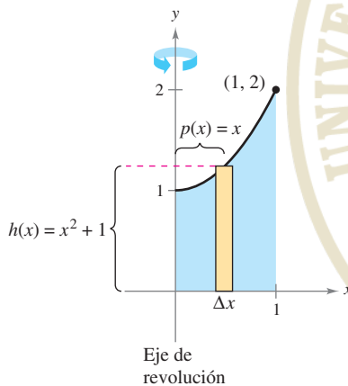
b) Método de las capas
