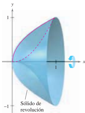
Sólido de revolución Figura 7.20
