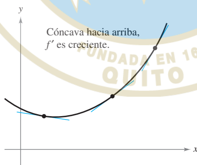
a) La gráfica de f se encuentra sobre sus rectas tangentes
