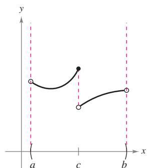
b) Discontinuidad inevitable o no removable
