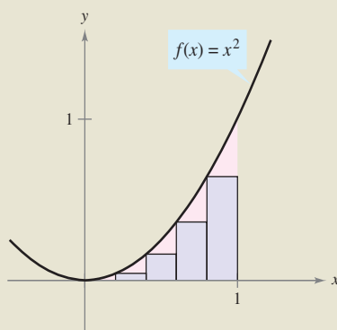
b) Rectángulos inscritos
