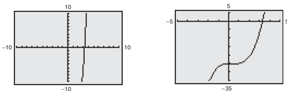
Visualizaciones en la pantalla de una herramienta de graficación de y = x^3 - x^2 - 25 Figura P.4
