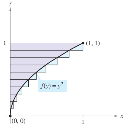
El área de la región acotada por la gráfica de f , el eje y para 0 \leq y \leq 1 es \frac{1}{3} . Figura 4.16
