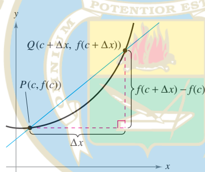
a) La recta secante que pasa por (c, f(c)) y (c + \Delta x, f(c + \Delta x))
