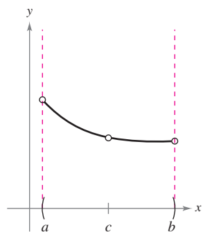
a) Discontinuidad evitable o removable
