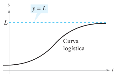
Notar que, como t \rightarrow \infty , y \rightarrow L Figura 6.17
