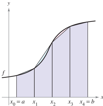
El área de la región puede aproximarse utilizando cuatro trapecios
