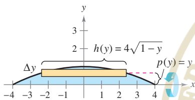
b) Método de las capas Figura 7.35
