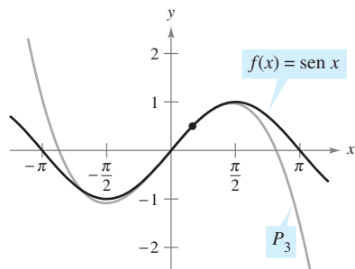
En la cercanía de (\pi/6, 1/2) , la gráfica de P_3 puede usarse para aproximar la gráfica de f(x) = \operatorname{sen} x Figura 9.16
