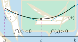
Mínimo relativo
