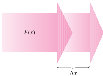
La magnitud de fuerza varía conforme cambia la posición de un objeto ( \Delta x )
