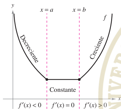
La derivada se relaciona con la pendiente de una función
