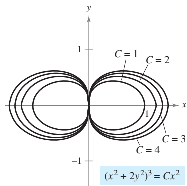
Solución general de (x^2 - y^2) dx + 3xy dy = 0
