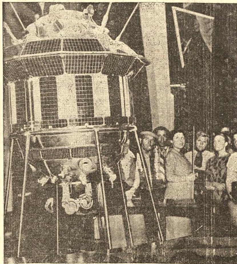
Modelo de la estación interplanetaria lanzada por el tercer cohete soviético y en cuyo interior se encuentran los equipos que permitieron fotografiar la parte oculta de la Luna.
