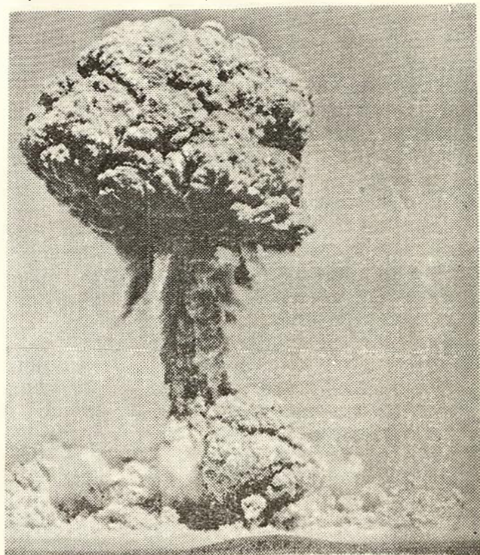
El cono radiactivo de una explosión atómica, se levanta como un signo fatídico de dolor, desolación y muerte.
