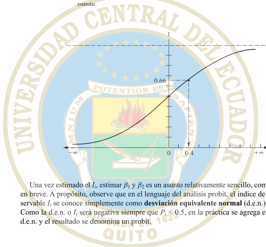
FIGURA 15.5 FDA normal.
